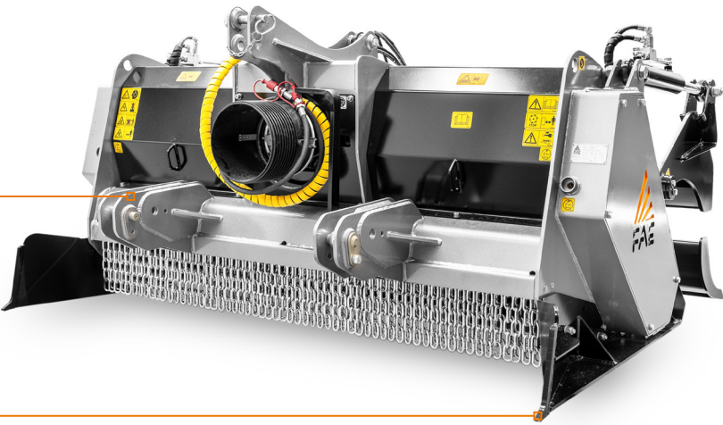
ペネトレーションスキッド 機械が土壌に より浸透しやすくなるよう後押し
