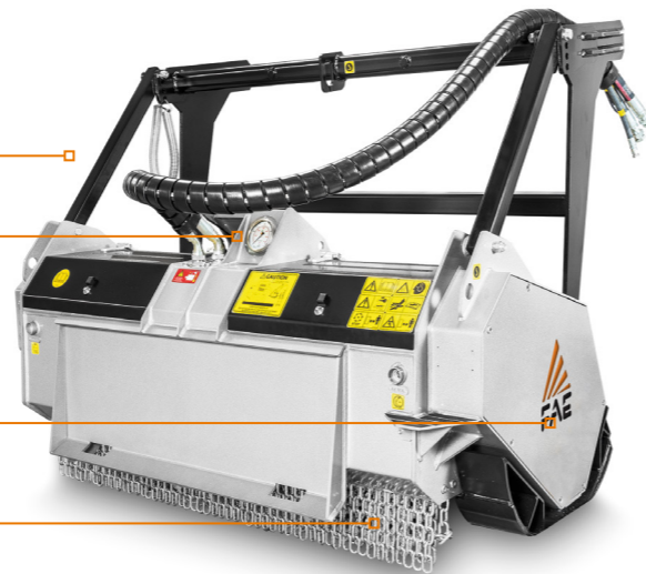
Sonic System (ソニックシステム) 油圧トランスミッションを管理する新しい自動インテリジェントシステムです。あらゆる条件 (UML/SSL/SONIC) 下で裁断マシン類の能力を最大に発揮させます
