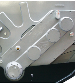
サイドギアボックス付き デュアルトランスミッション ローターへの動力伝達を増大
